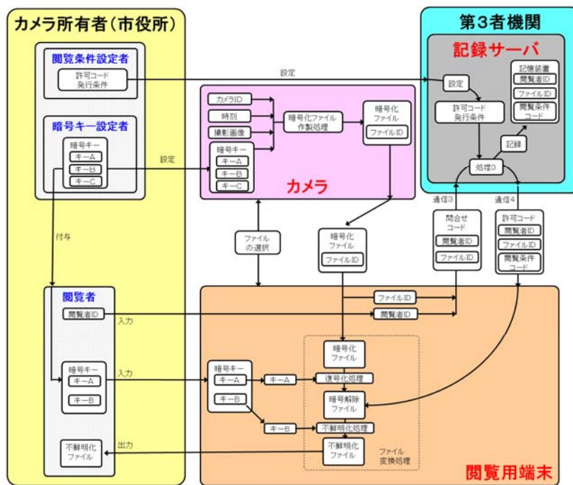
図2 閲覧行動の記録の仕組み：カメラ＝閲覧装置＝記録サーバ間のデータのやり取り
